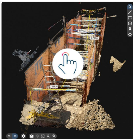
Mapiranje podzemnih radova
