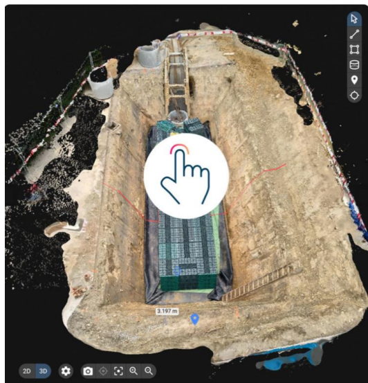
Monitoriranje iskopa i betoniranja
